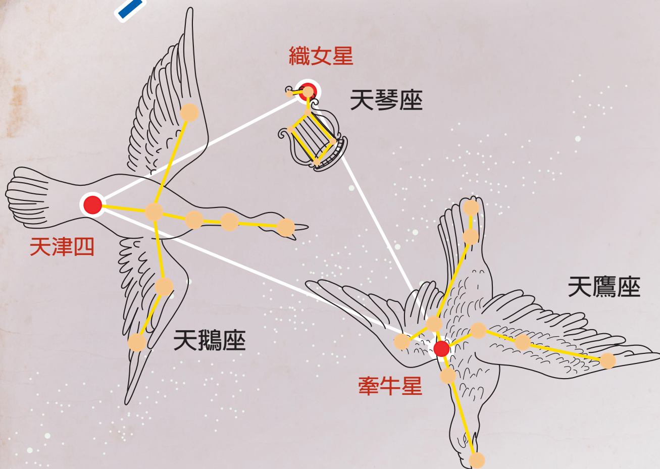
▲ 牽牛、織女星座示意圖（夏季大三角）
