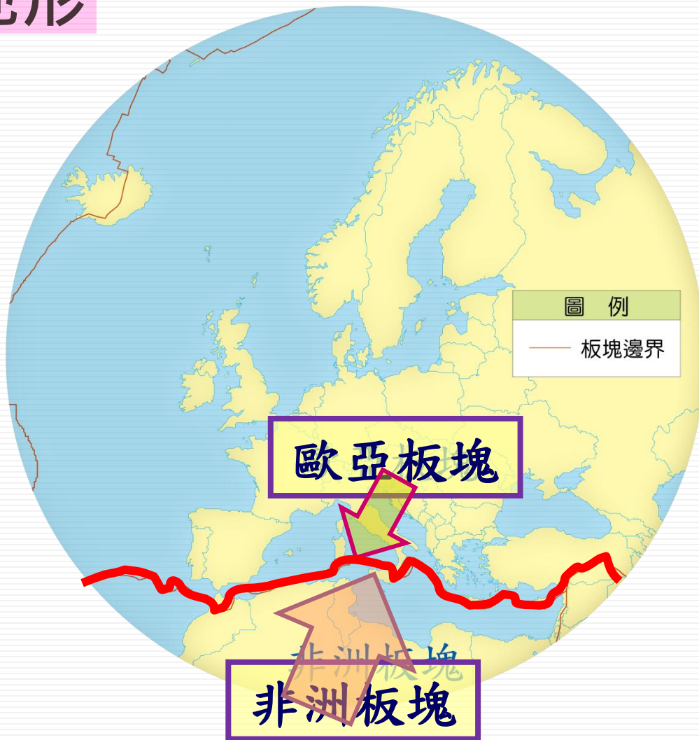
圖1-1-1 歐洲板塊分布圖
