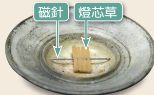
▲圖3-3-13 指南針復原模型 / 以磁石磨擦鐵針，再用燈芯草包覆後放在盛水的碗中，即有指南的效果。指南針運用於航海技術，有助於對外貿易的發展。
