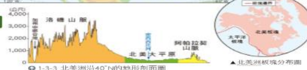
1-3-3 北美洲沿40°N的地形剖面圖
